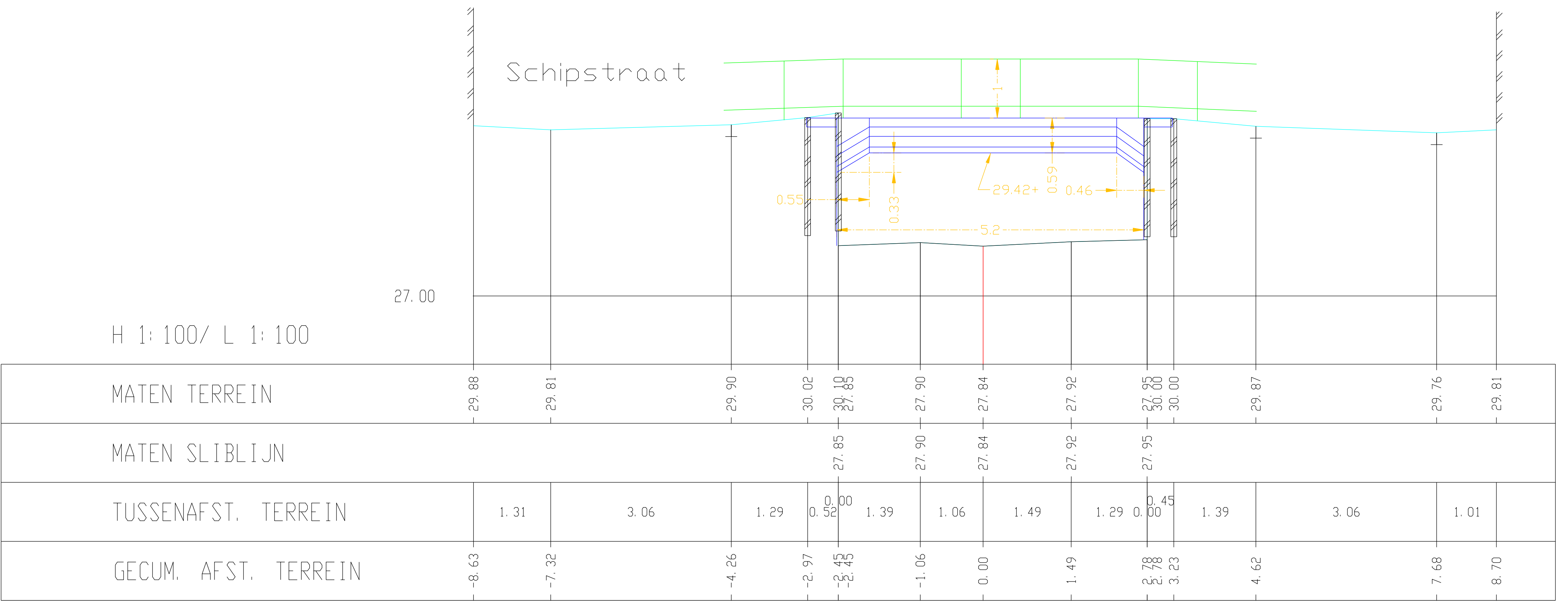
Kleine Gete, Dwarsprofiel 096
