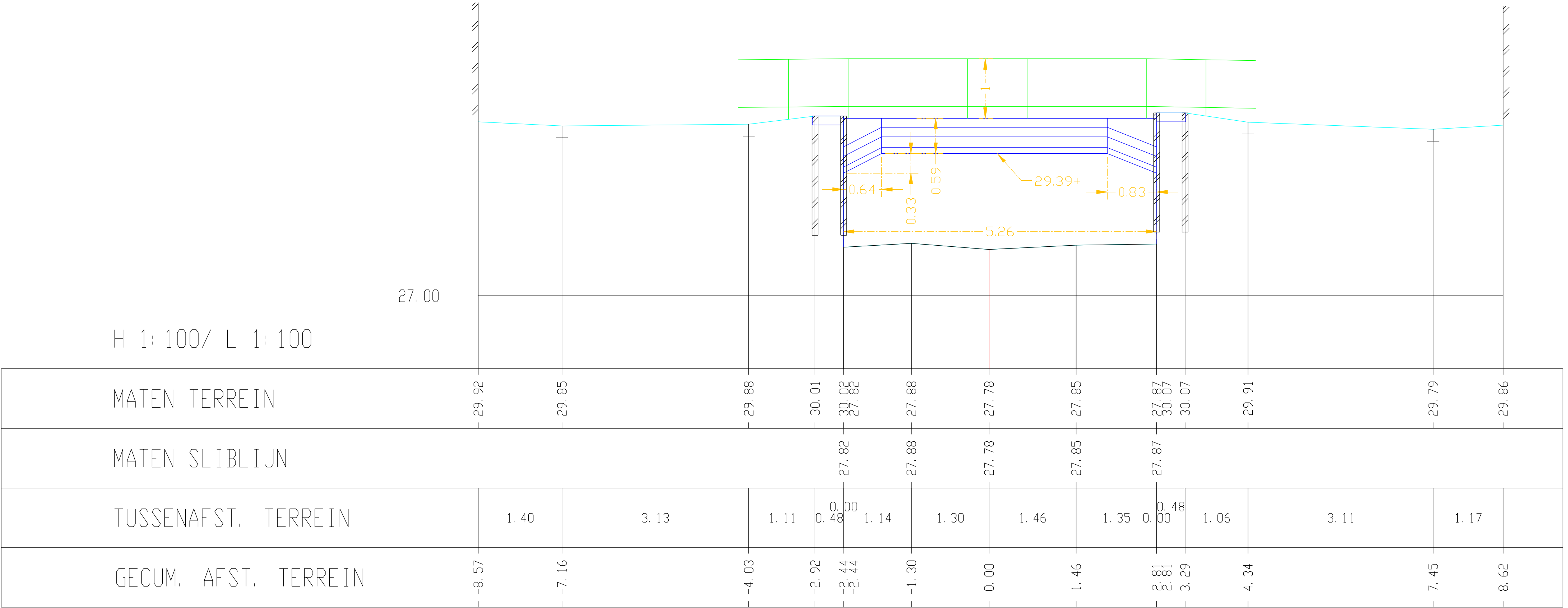
Kleine Gete, Dwarsprofiel 098
