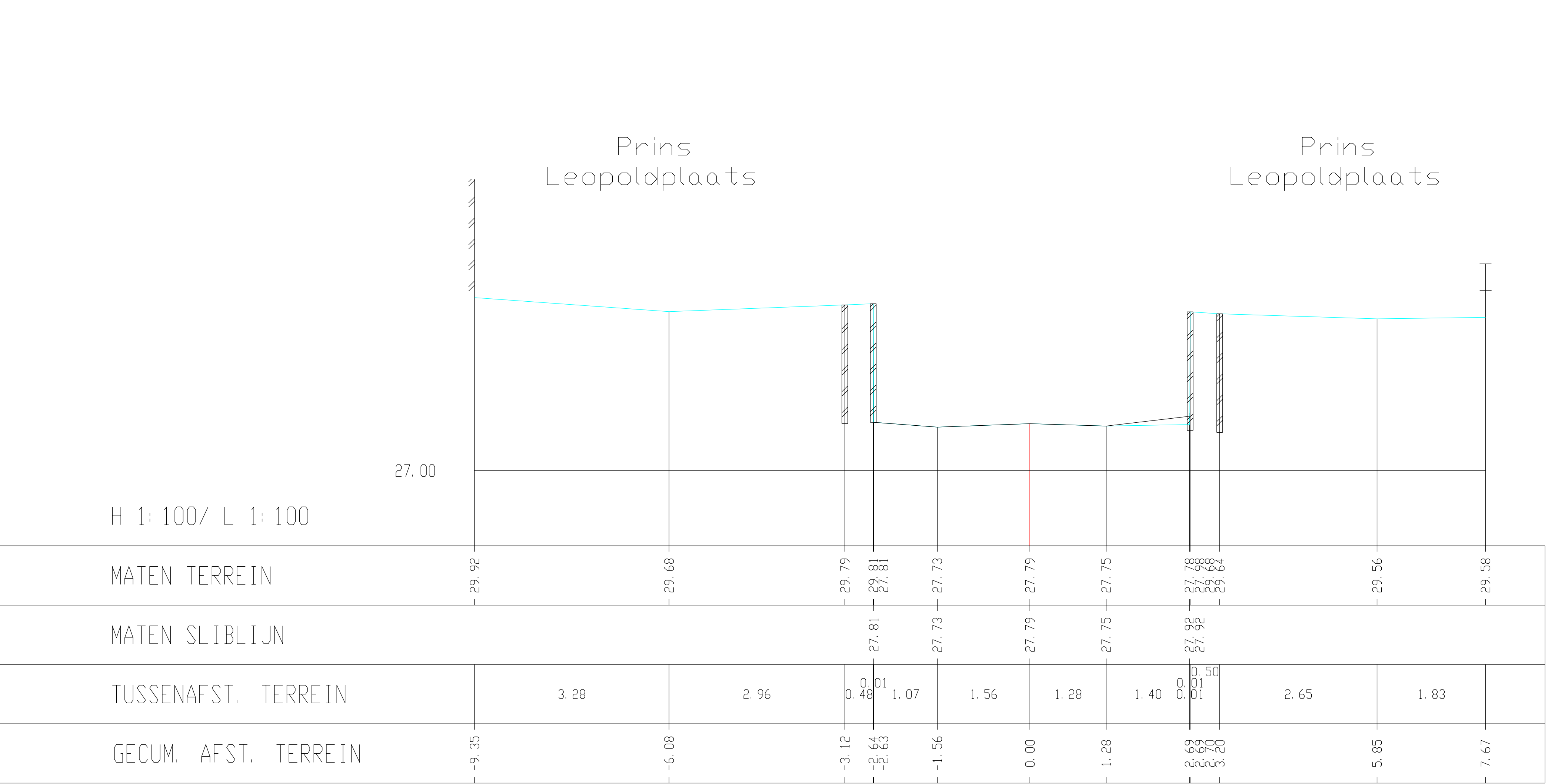
Kleine Gete, Dwarsprofiel 099
