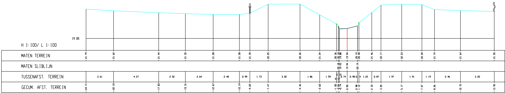
Leugebeek, Dwarsprofiel K018
