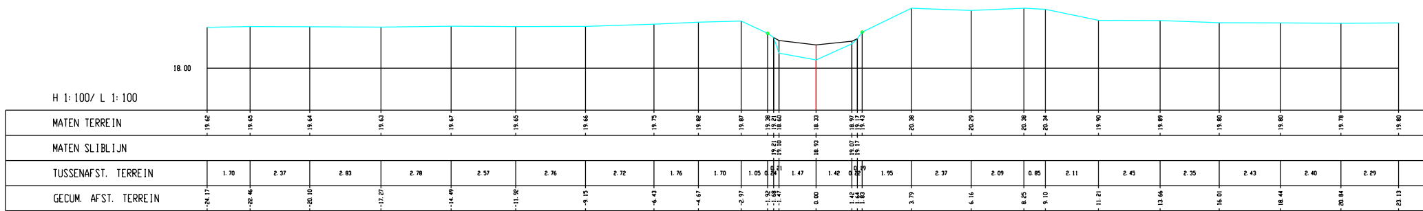
Leugebeek, Dwarsprofiel K002
