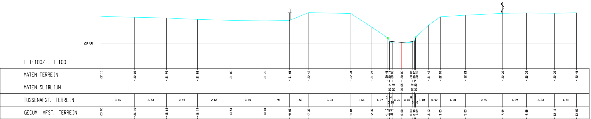
Leugebeek, Dwarsprofiel K020
