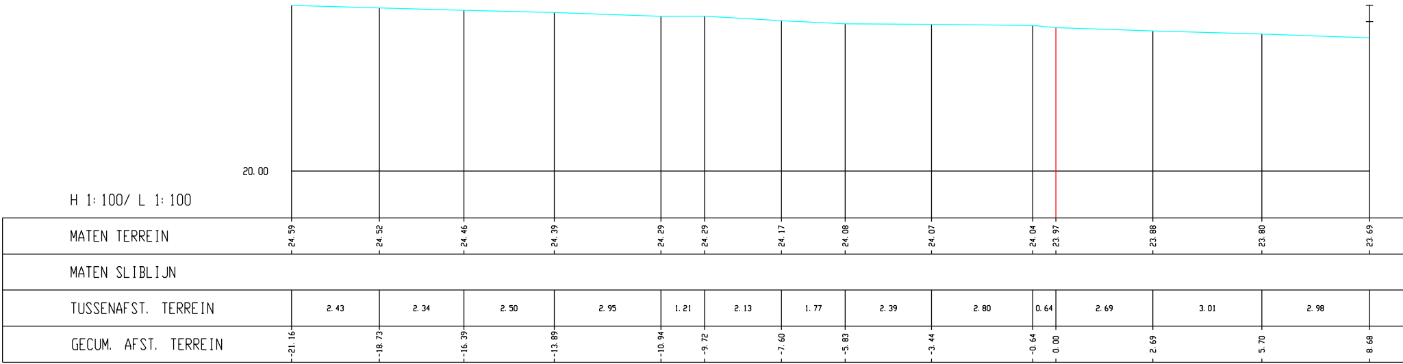
Leugebeek, Dwarsprofiel K027
