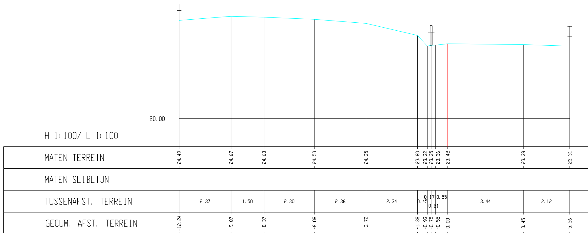
Leugebeek, Dwarsprofiel K029
