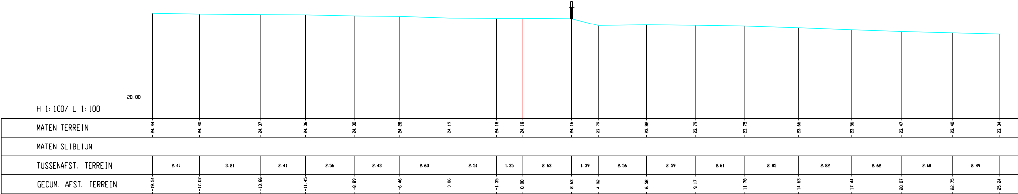
Leugebeek, Dwarsprofiel K032
