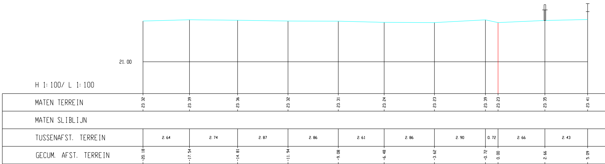
Leugebeek, Dwarsprofiel K037
