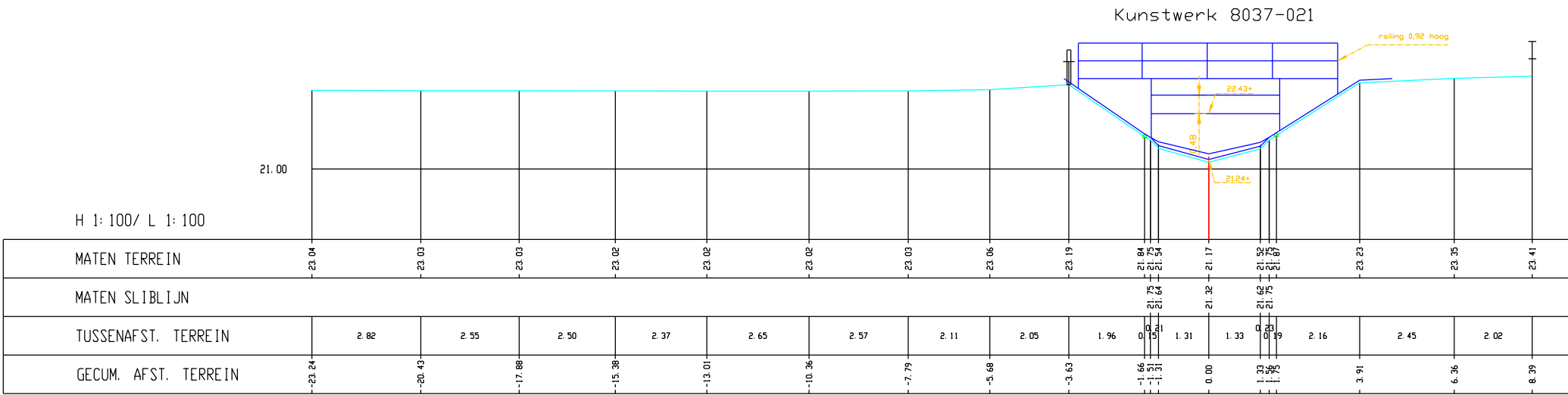
Leugebeek, Dwarsprofiel K039
