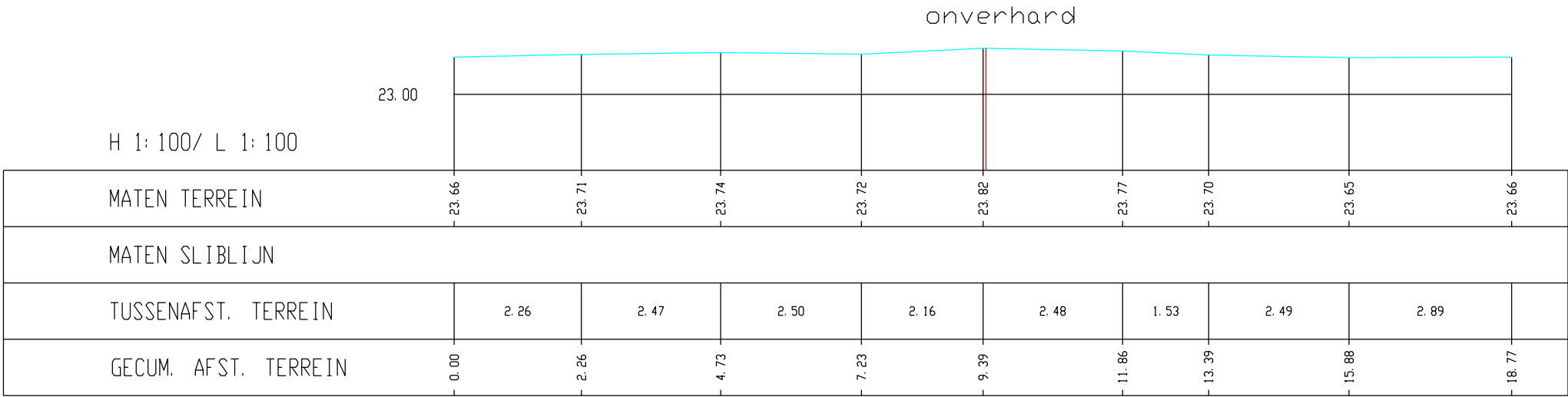
Leugebeek, Dwarsprofiel K045
