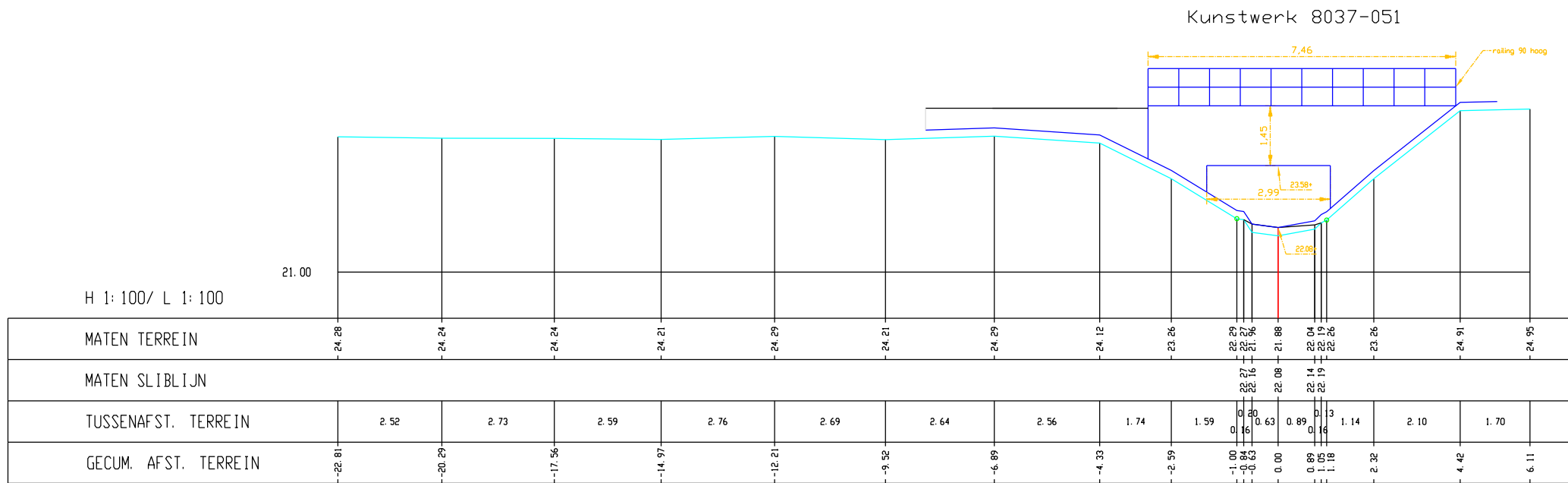
Leugebeek, Dwarsprofiel K054
