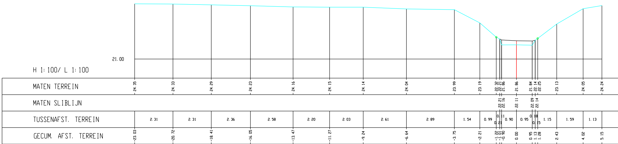
Leugebeek, Dwarsprofiel K056
