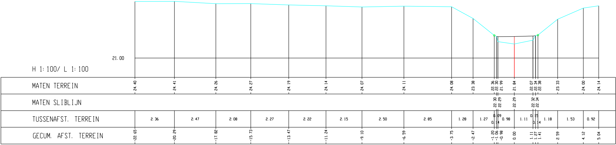
Leugebeek, Dwarsprofiel K057
