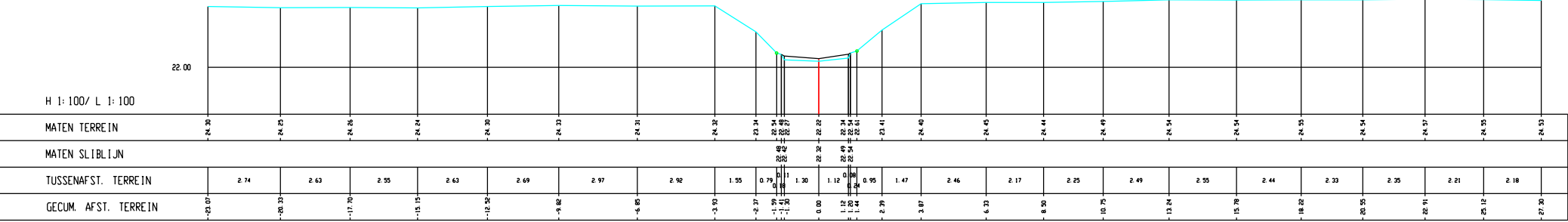
Leugebeek, Dwarsprofiel K063
