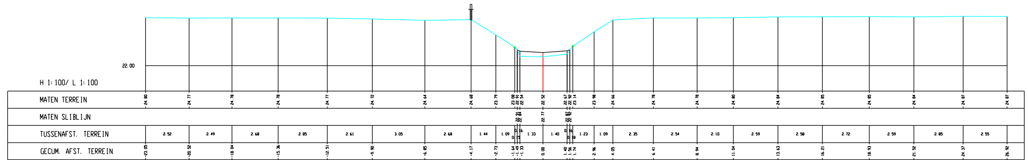
Leugebeek, Dwarsprofiel K079
