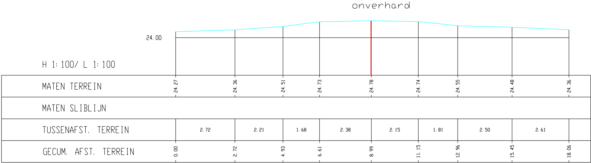
Leugebeek, Dwarsprofiel K081
