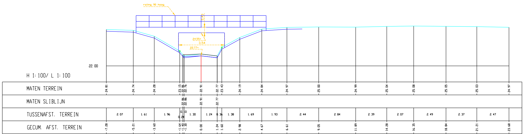
Leugebeek, Dwarsprofiel K086
