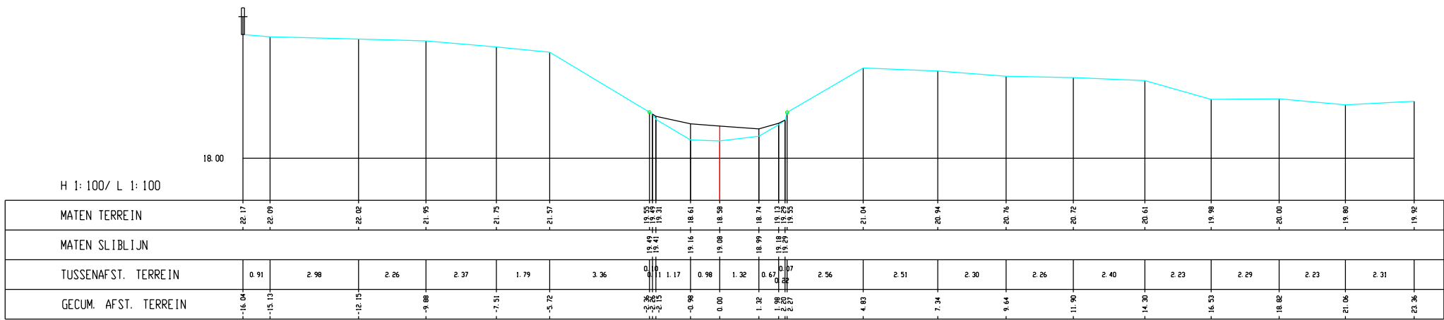
Leugebeek, Dwarsprofiel K009
