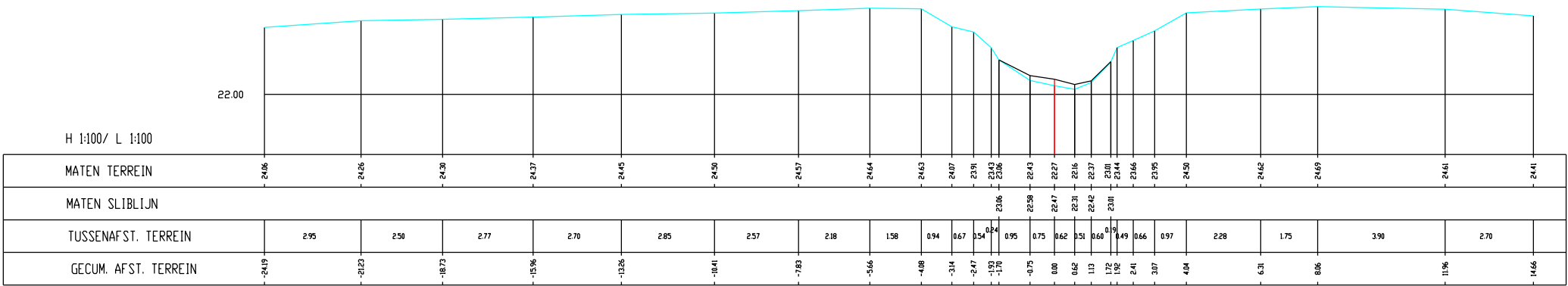
Mangelbeek, Dwarsprofiel k100
