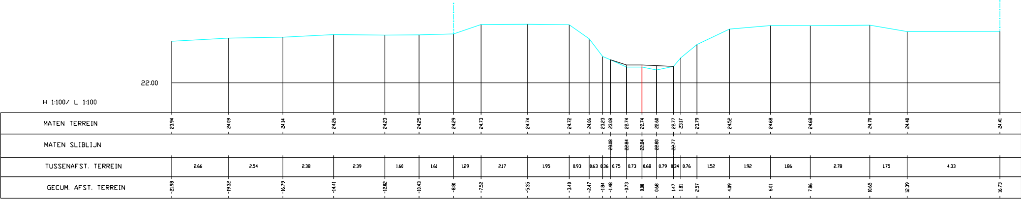
Mangelbeek, Dwarsprofiel k107
