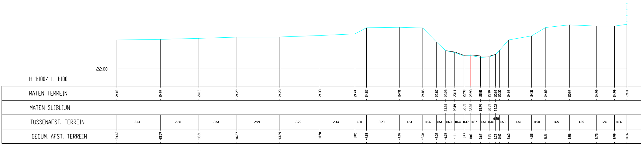
Mangelbeek, Dwarsprofiel k112
