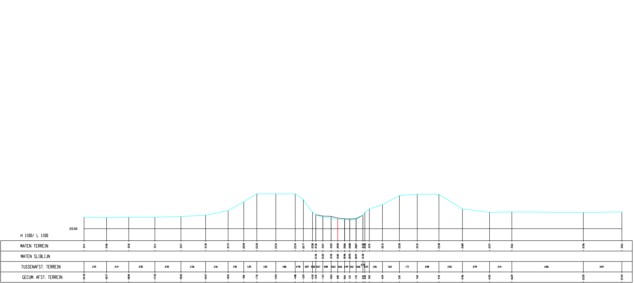
Mangelbeek, Dwarsprofiel k15
