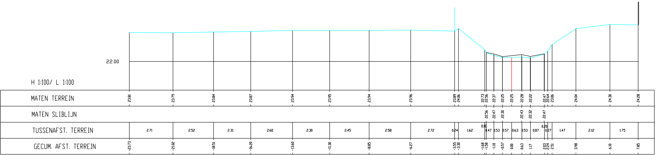
Mangelbeek, Dwarsprofiel k73
