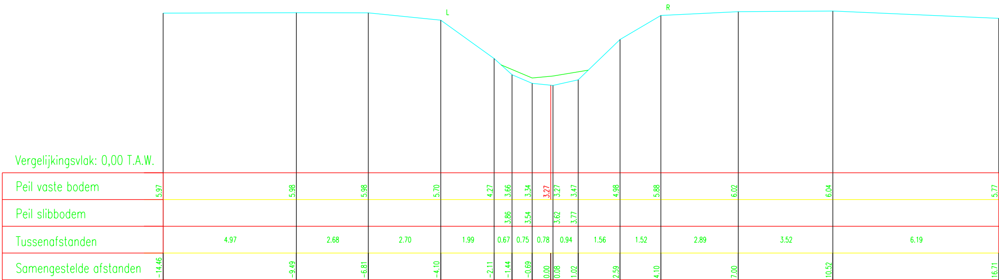
DWARSPROFIEL 56 Schaal 1/100
