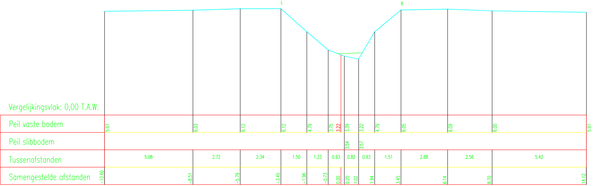
DWARSPROFIEL 4 Schaal 1/100
