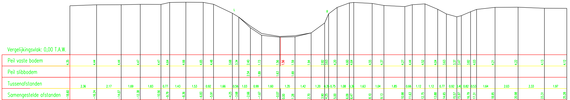
DWARSPROFIEL 12A Schaal 1/100
