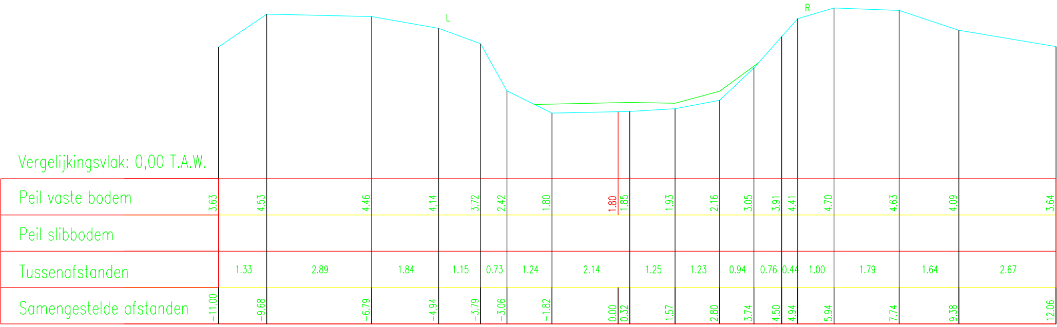
DWARSPROFIEL 40 Schaal 1/100
