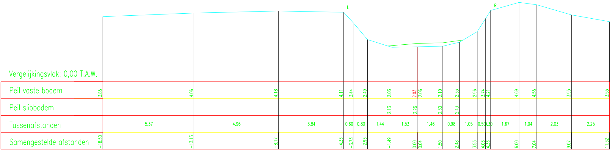
DWARSPROFIEL 42 Schaal 1/100
