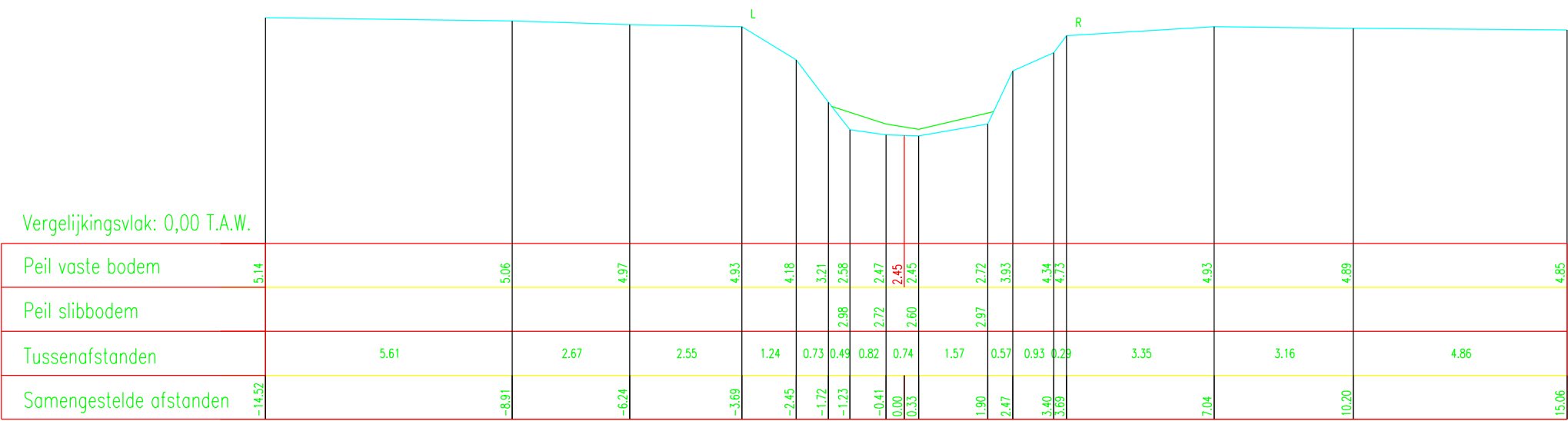
DWARSPROFIEL 28 Schaal 1/100
