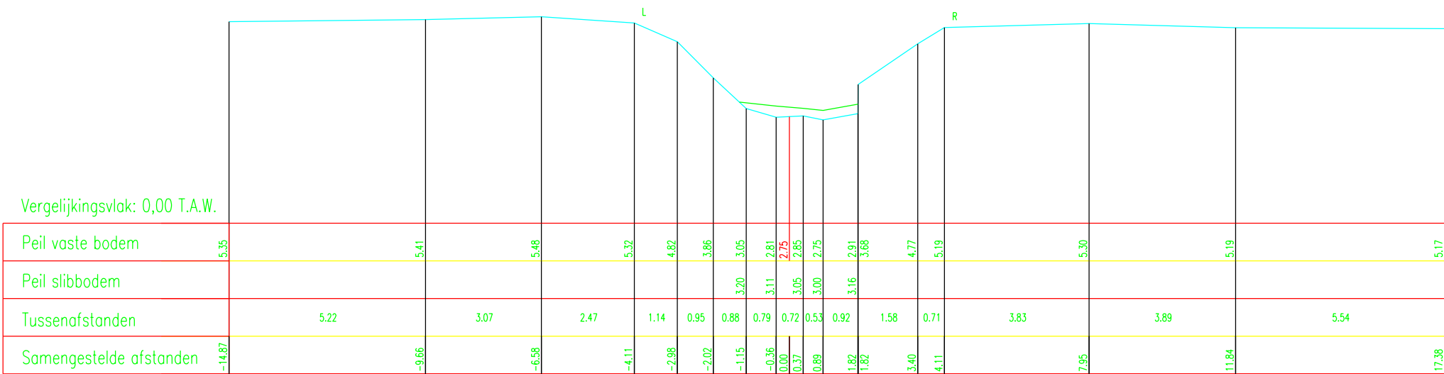
DWARSPROFIEL 37 Schaal 1/100
