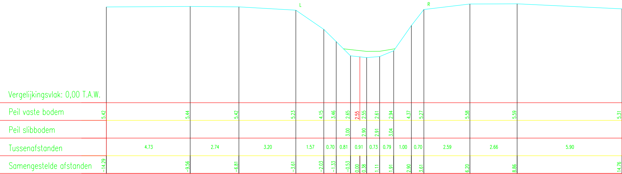
DWARSPROFIEL 41 Schaal 1/100
