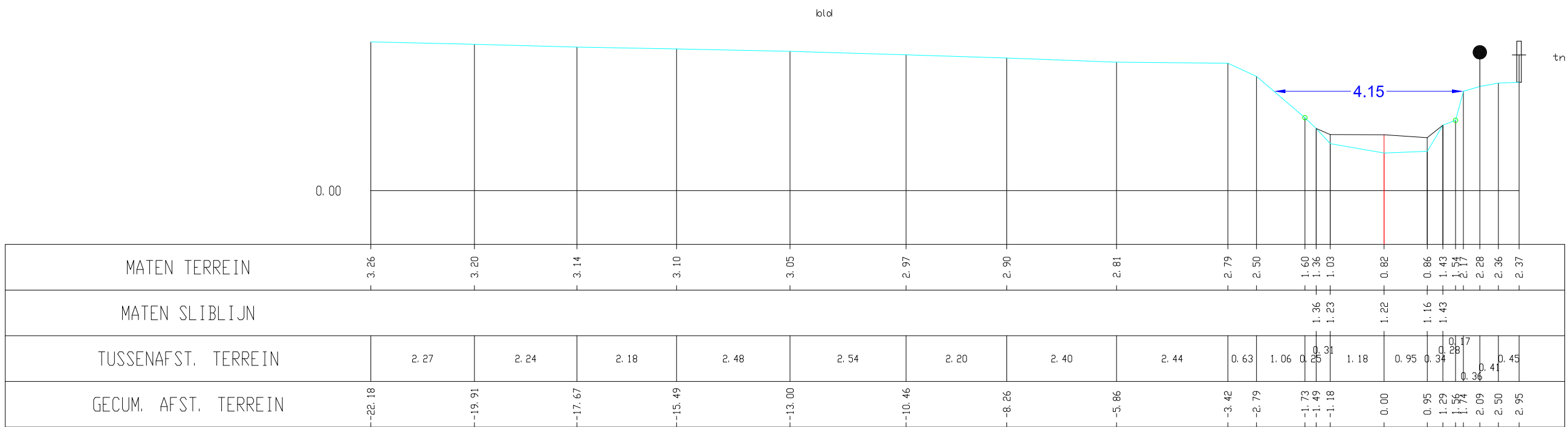
O8371_VHAG_3027, Dwarsprofiel 5
