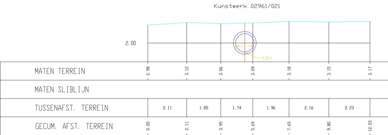
Molenkreek 02961/08376, Dwarsprofiel 043
