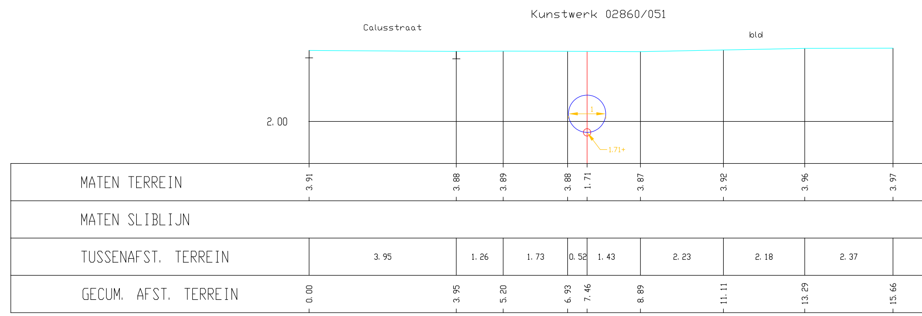
O8383_2860, Dwarsprofiel 012
