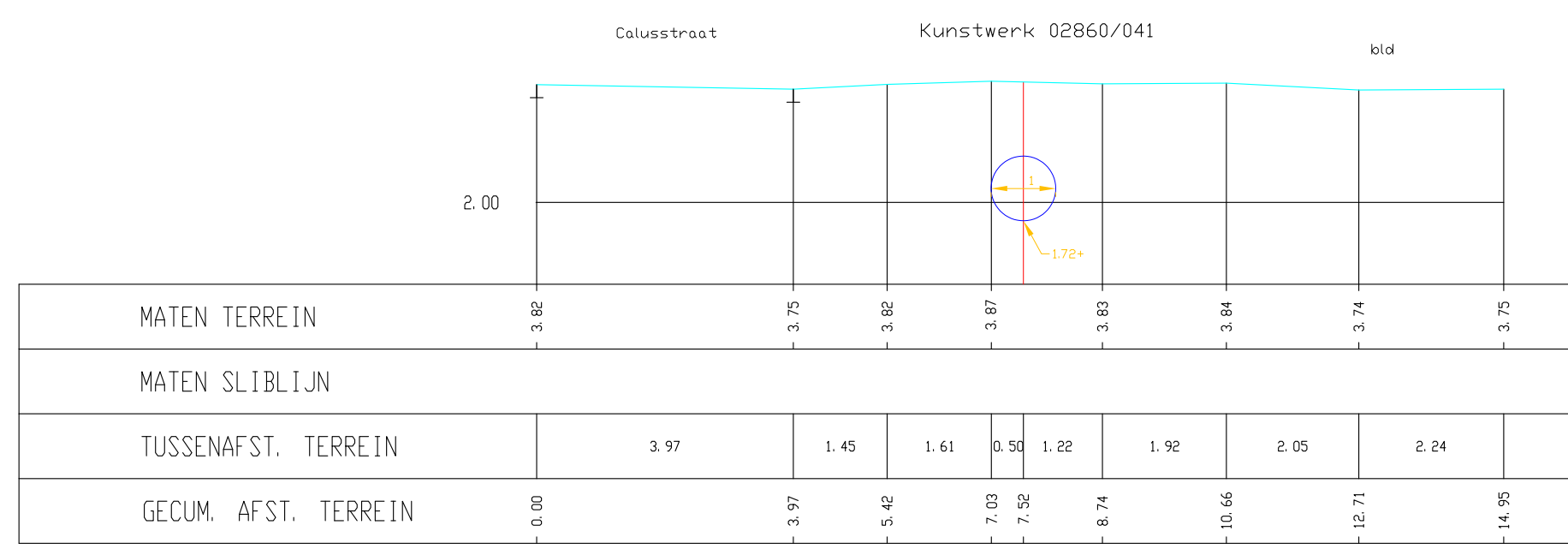
O8383_2860, Dwarsprofiel 021
