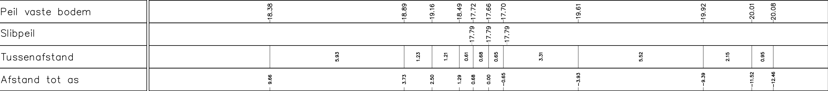
Dwarsprofiel 25 Vergelijkingsvlak 16.00 m T.A.W. 7+14.60
