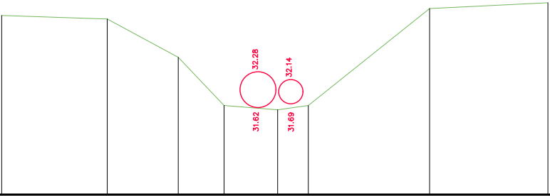
DWARSPROFIEL Vergelijkingsvlak 30.00 m T.A.W.
