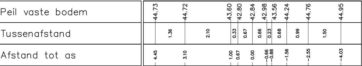
Dwarsprofiel 8 Vergelijkingsvlak 42.00 m T.A.W. 2+80.07
