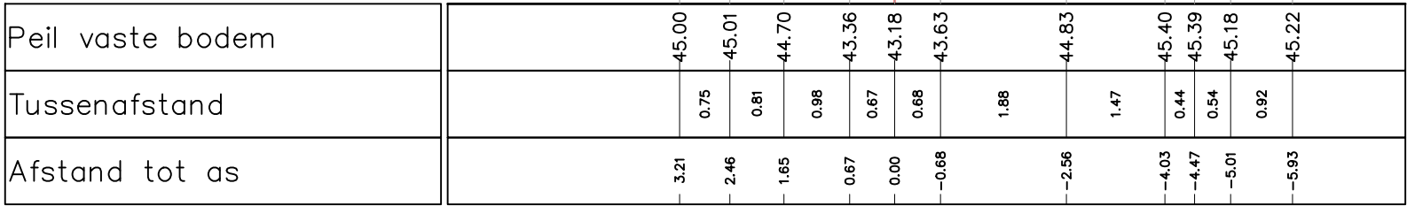
Dwarsprofiel 10 Vergelijkingsvlak 42.00 m T.A.W. 3+84.13
