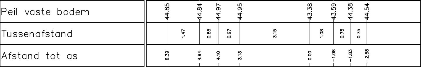
Dwarsprofiel 15 Vergelijkingsvlak 42.00 m T.A.W. 6+91.42
