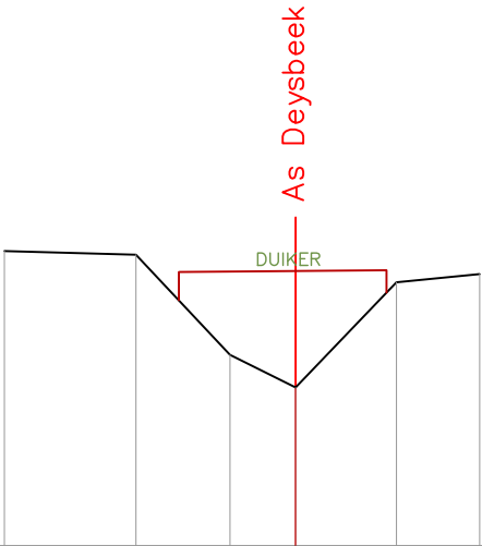
Dwarsprofiel 19 Vergelijkingsvlak 42.00 m T.A.W. 8+91.26
