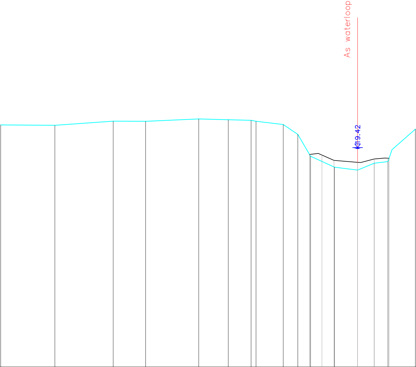
Dwarsprofiel 149 Vergelijkingsvlak 10.00 m T.A.W. Afstand op as 65+00.38
