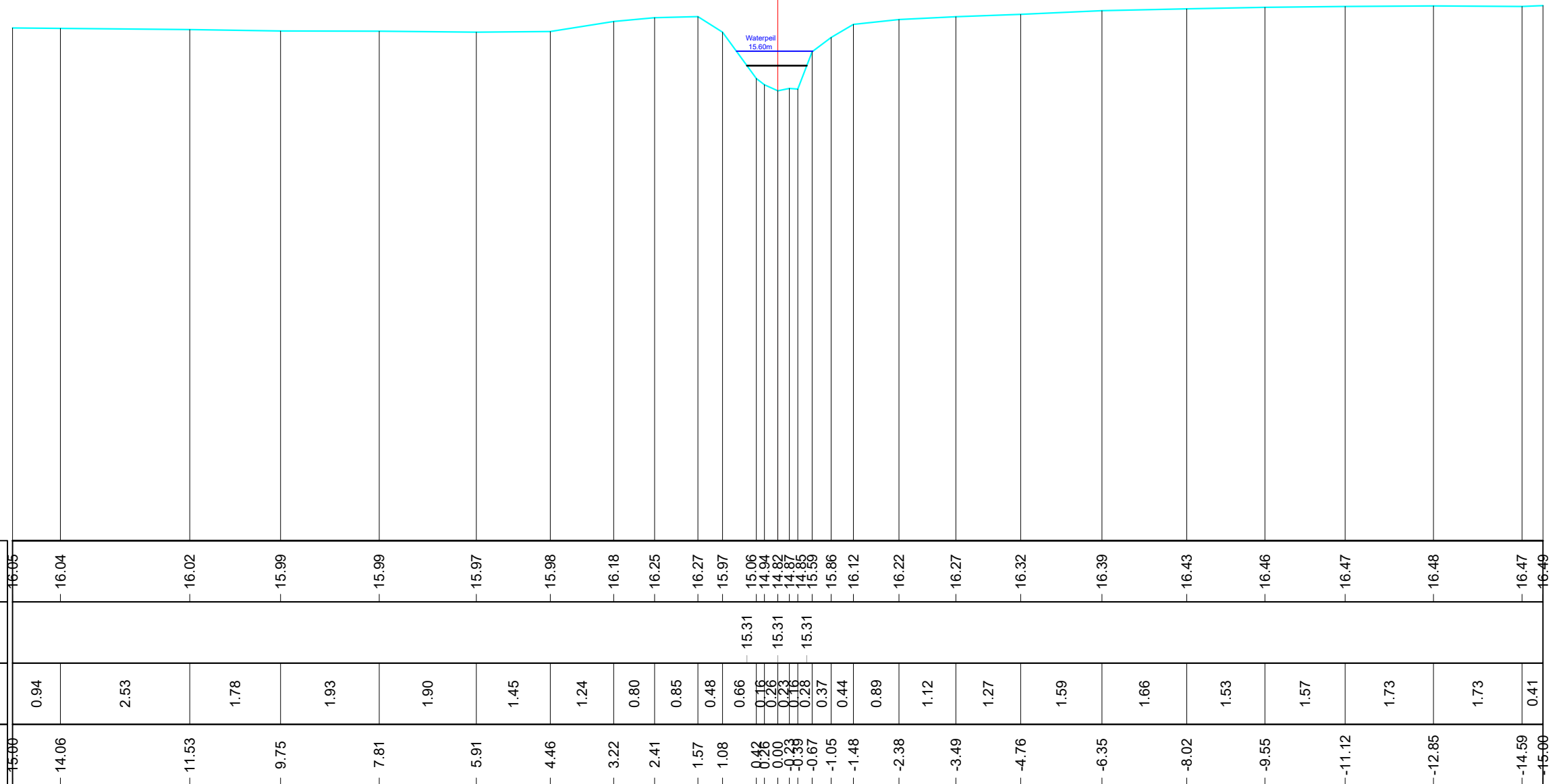
Dwarsprofiel 39 Vergelijkingsvlak 6.00 m T.A.W. Afstand op as 659.18m
