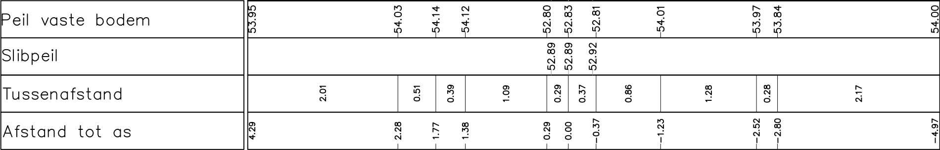
Dwarsprofiel 7 Vergelijkingsvlak 52.00 m T.A.W. 2+81.46
