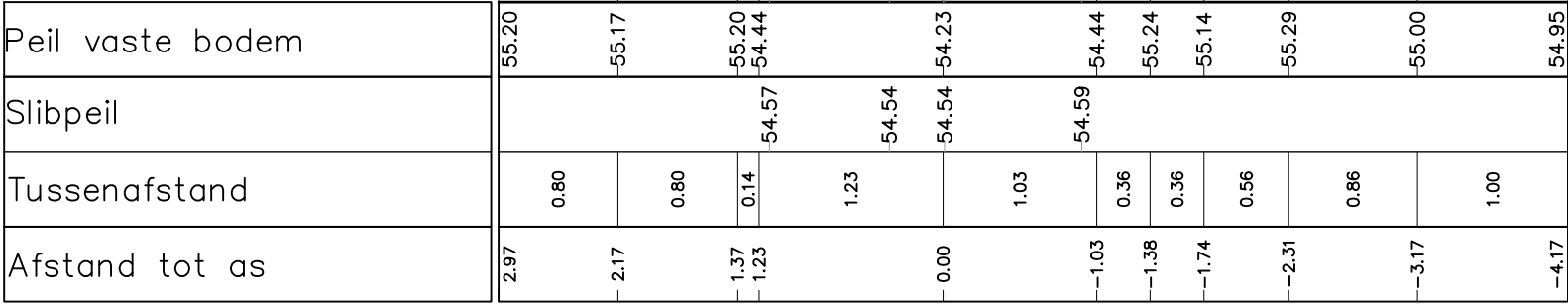
Dwarsprofiel 9 Vergelijkingsvlak 54.00 m T.A.W. 3+76.67
