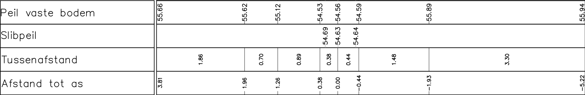
Dwarsprofiel 11 Vergelijkingsvlak 54.00 m T.A.W. 4+58.70
