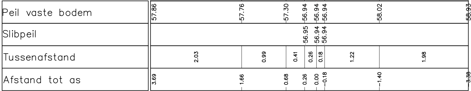
Dwarsprofiel 17 Vergelijkingsvlak 56.00 m T.A.W. 7+53.49
