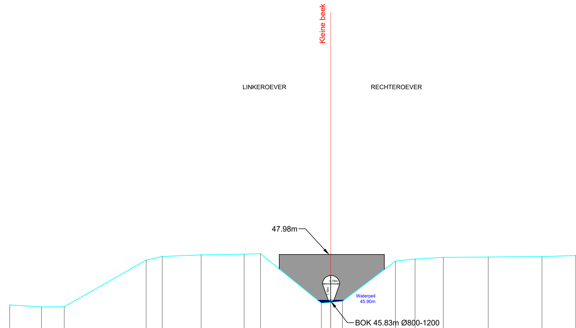
Dwarsprofiel 1 Vergelijkingsvlak 44.00 m T.A.W. Afstand op as 025.28m
